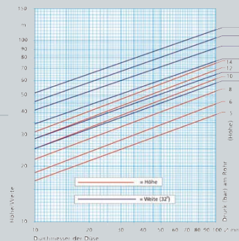
Wurfweite und -höhe von Wasser-Strahlrohren
