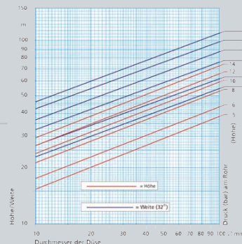
Wurfweite und -höhe von Schaum-/Wasser-Strahlrohren
