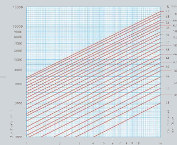
Durchsatz von Wasser- und Schaum-/Wasser-Strahlrohren
