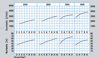
Leistungsdiagramm Mehrzweckdüse
