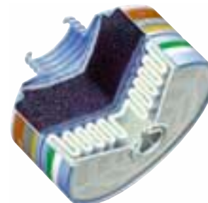
Kombifilter
